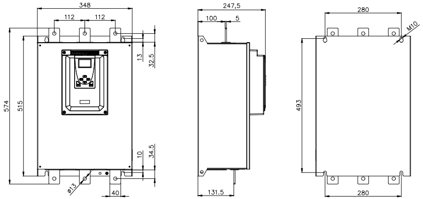
图 2.5 132kW~200kW 外形安装尺寸图 (380V)
