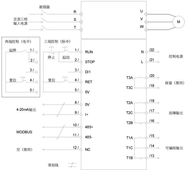
图 3.2 标准接线图
