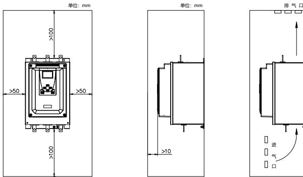
图 3.1 安装要求示意图
