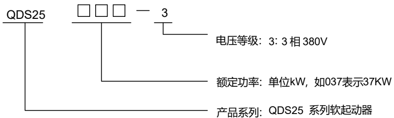
图 2.2 软起动机型号说明示意图
