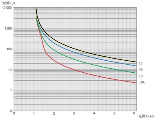
图 5.7 电机过载保护级别特性
