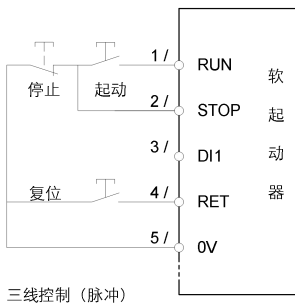
(a) 三线控制相关端子接线
