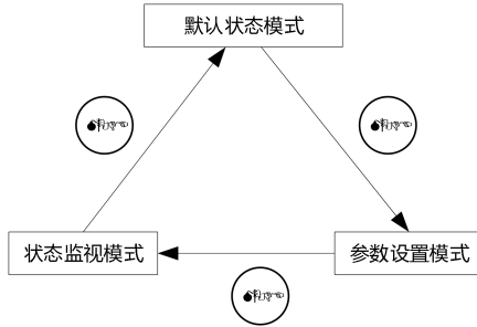
图 4.2 软起动器模式切换示意图
