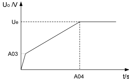
图 5.1 电压斜坡起动示意图
