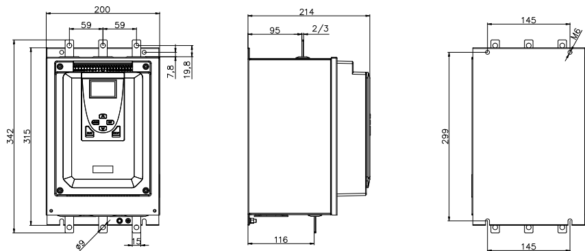
图 2.3 5.5kW~55kW 外形安装尺寸图 (380V)
