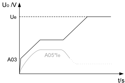
图 5.3 电压斜坡+限流启动示意图
