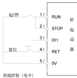
(b) 两线控制相关端子接线
