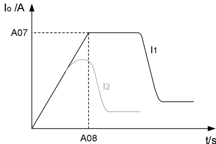
图 5.5 电流斜坡起动示意图
