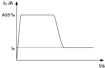
图 5.2 电流限流启动示意图
