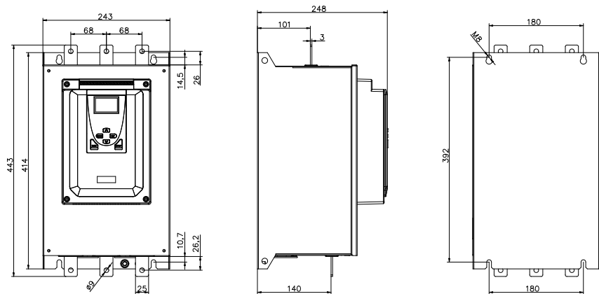
图 2.4 75kW~115kW 外形安装尺寸图 (380V)
