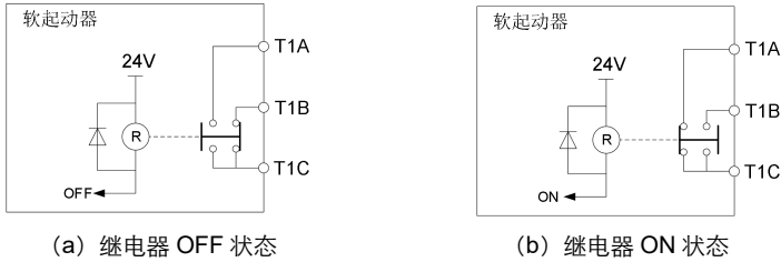
图 5.8 继电器状态说明
