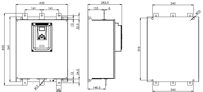
图 2.6 250kW~320kW 外形安装尺寸图 (380V)
